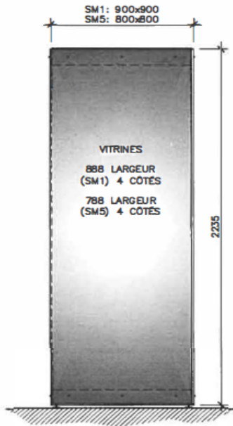
ÉLÉVATION TYPIQUE VITRINE SM1 & SM5 Echelle: 1=15
