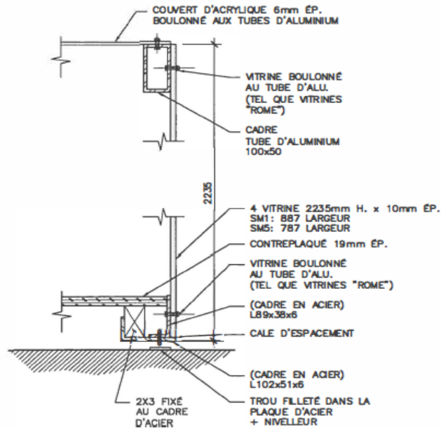
COUPE TYPIQUE Echelle: 1=5
